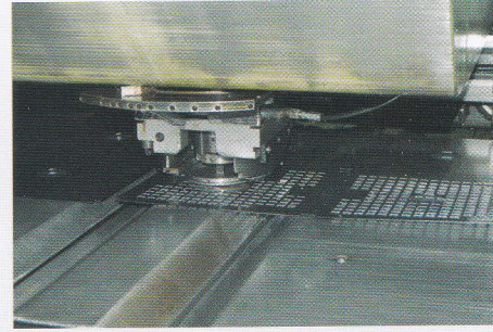
Stancolás, perforálás
