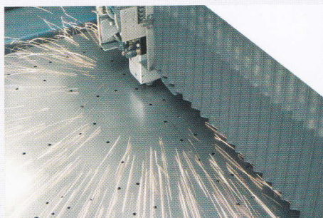
Lézervágás
