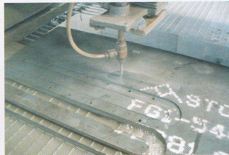
Vízzel vágás
